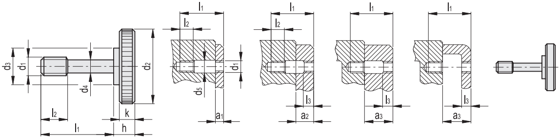
Tipi di montaggio
